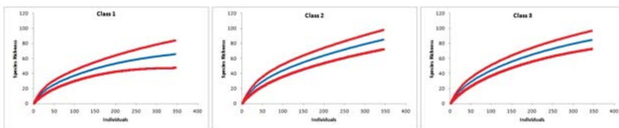
Figura 2 – Riqueza estimada entre as classes de tamanhos 1, 2 e 3 das plantas em fragmento de FES em Sorocaba, SP. A curva de rarefação extrapolada foi calculada no EstimateS, considerando 345 indivíduos. As curvas em azul representam a riqueza média e as curvas em vermelho, o intervalo de confiança de 95% (Classes: 1, pelo menos 2 pares de folhas e \leq 100 cm de altura; 2, > 100 cm de altura e circunferência em nível do solo \leq 15 cm; e 3, circunferência à altura do peito \geq 15 cm).
